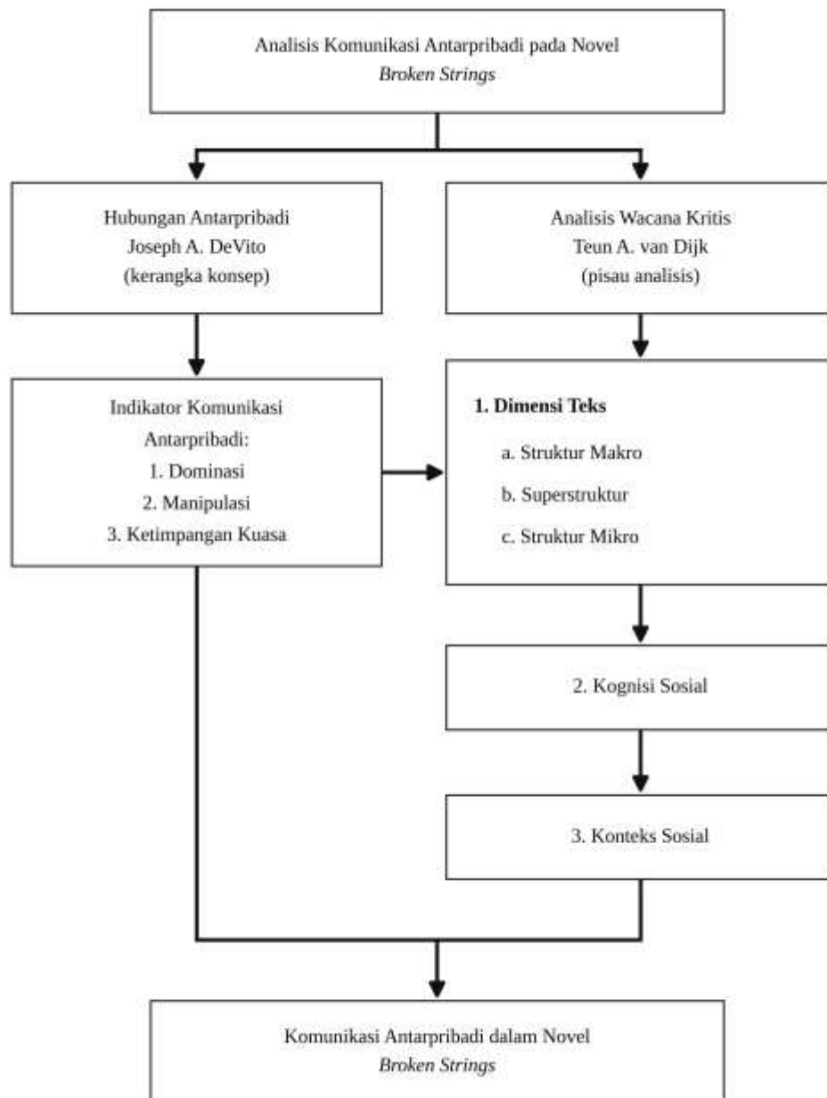
Gambar 2.2. Kerangka Pemikiran
