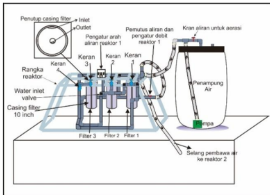
Gambar 1. Reaktor 1
