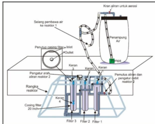
Gambar 2. Reaktor 2
