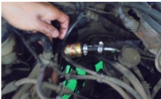
Gambar 5. Pemasangan Ionizer BBM pada Sampel Mobil
