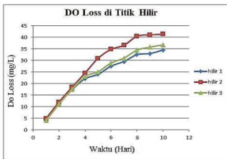
Gambar 5. DO Loss Segmen Hilir
