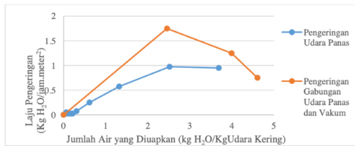
Gambar 8 Grafik kecepatan pengeringan dengan massa bahan awal 200 gram
