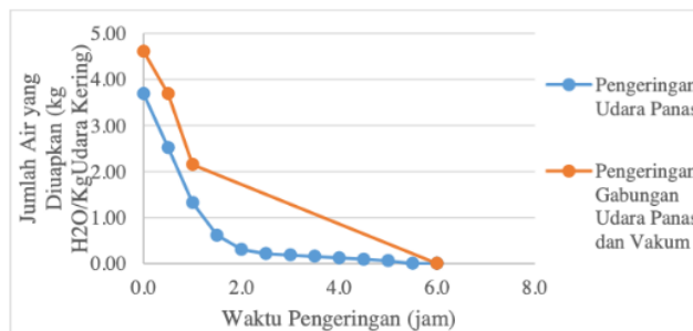
Gambar 7 Grafik hubungan jumlah air yang diuapkan dengan waktu pengeringan dengan massa bahan awal 200 gram
