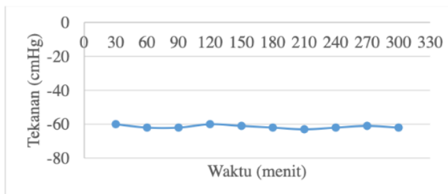
Gambar 6 Grafik pengukuran tekanan di ruang pengering
