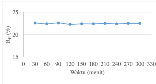
Gambar 5 Grafik pengukuran R H di ruang pengering
