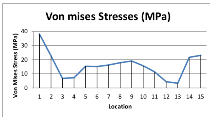
Gambar 7. Result Von mises Stress
