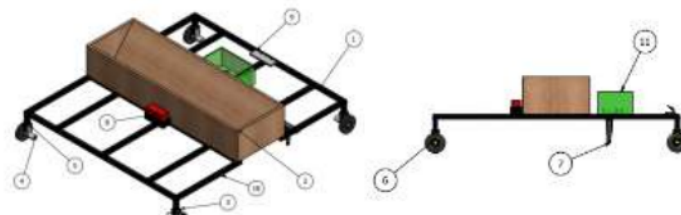
Gambar 1. Rancangan Mobil Robot Penanam Bibit Kangkung
