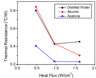
Fig. 11 Thermal resistances
