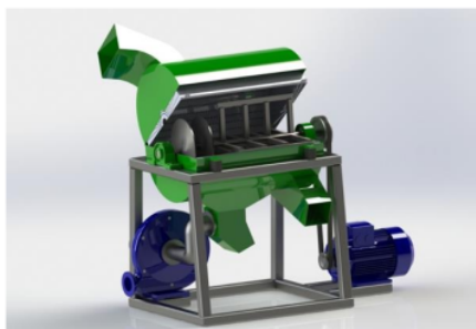
Gambar 9. Rangkaian Mesin Peorontok
