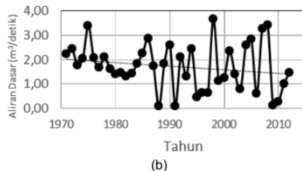
Gambar 2. (a) Peningkatan nilai koefisien limpasan dan (b) Penurunan nilai aliran dasar
