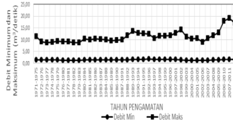
Gambar 3. Moving average debit maksimum dan minimum tahunan
