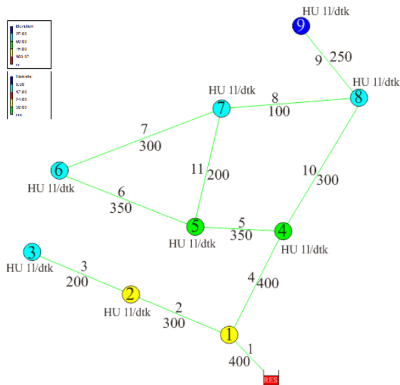
Gambar 2. Jaringan pipa distribusi hasil simulasi Epanet
