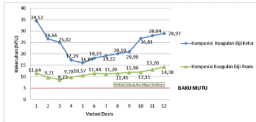
Gambar 5. Hubungan Variasi Komposisi Koagulan Dengan Kekeruhan 100 NTU
