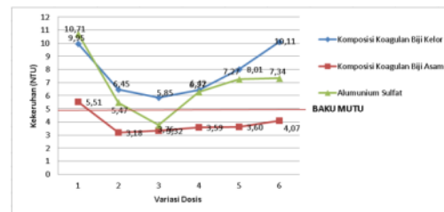
Gambar 9. Penyisihan kekeruhan air sungai terhadap variasi dosis koagulan
