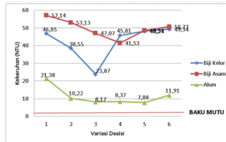
Gambar 4. Hubungan Variasi Dosis Koagulan Dengan Kekeruhan 1000 NTU
