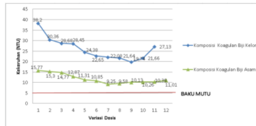
Gambar 8. Hubungan Variasi Komposisi Koagulan Dengan Kekeruhan 1000 NTU
