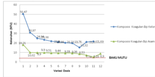
Gambar 7. Hubungan Variasi Komposisi Koagulan Dengan Kekeruhan 600 NTU
