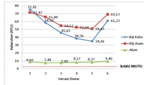
Gambar 3. Hubungan variasi dosis koagulan dengan kekeruhan 600 NTU
