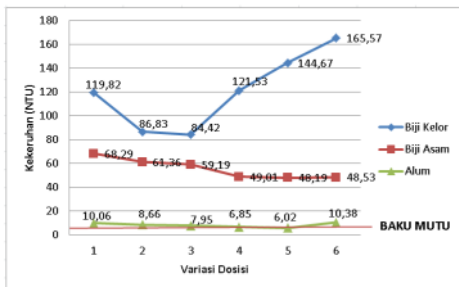
Gambar 2. Hubungan Variasi Dosis Koagulan Dengan Kekeruhan 500 NTU
