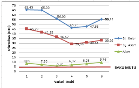
Gambar 1. Hubungan Variasi Dosis Koagulan Dengan Kekeruhan 100 NTU
