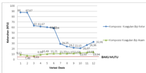
Gambar 6. Hubungan Variasi Komposisi Koagulan Dengan Kekeruhan 500 NTU
