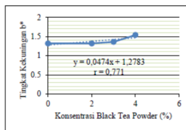
Gambar 5 Grafik korelasi antara konsentrasi black tea powder dengan Tingkat Kekuningan ( b^* )
