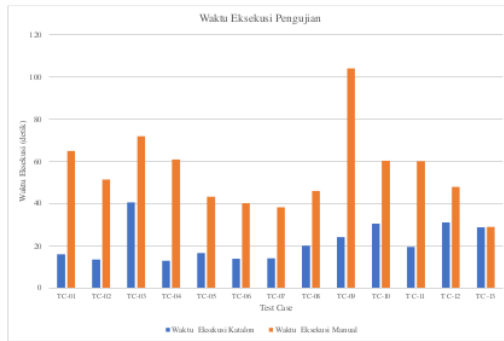
Gambar 20 Grafik waktu pengujian
