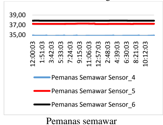
Gambar. 4.5. Distribusi Temperatur hari-3
