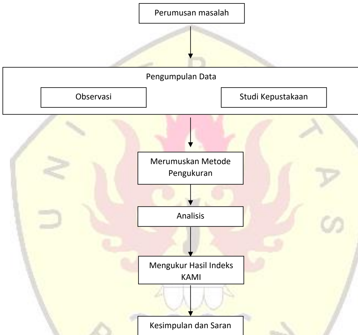
Gambar 1 1 Metodologi Penelitian
