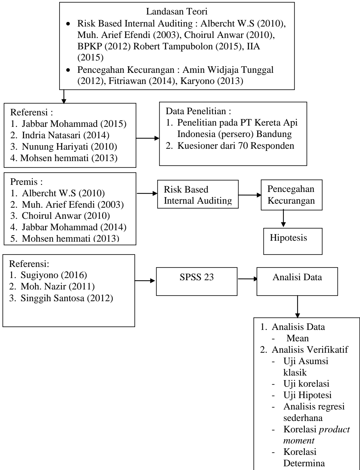
Gambar 2.2 Kerangka Pemikiran
