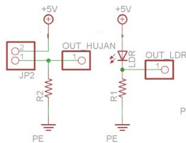
Gambar 2.15 Skematik Rangkaian Sensor Hujan
