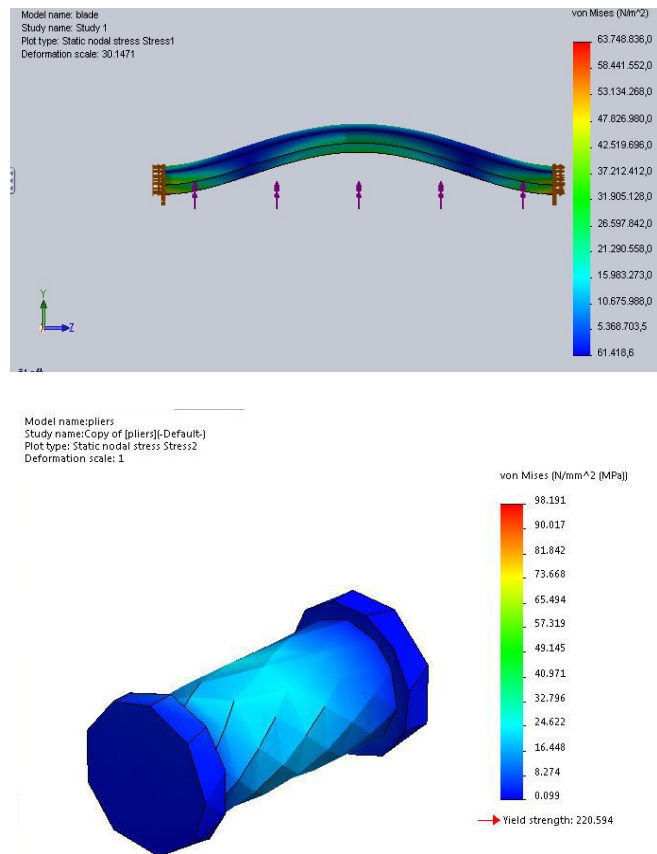
Gambar 2.21 Contoh Benda Kerja yang Telah Dilakukan Solidwork Simulation
