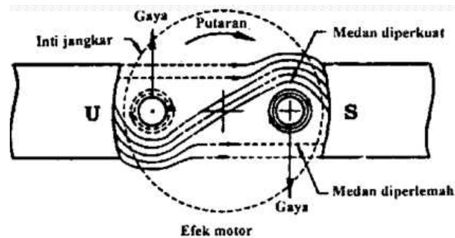
Gambar 2.11 Skematis Prinsip Kerja Motor DC
