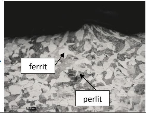
Daerah Struktur Mikro pada sprocket lokal kondisi As it is (340x pembesaran) Etsa Nital
