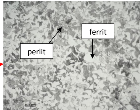
Daerah Struktur Mikro pada sprocket lokal kondisi As it is (170x pembesaran) Etsa Nital
