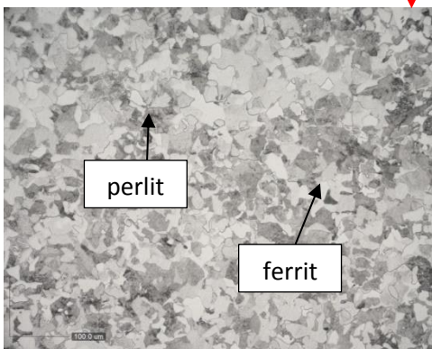
Daerah Struktur Mikro pada sprocket lokalkondisi As it is (170x pembesaran) Etsa Nital
