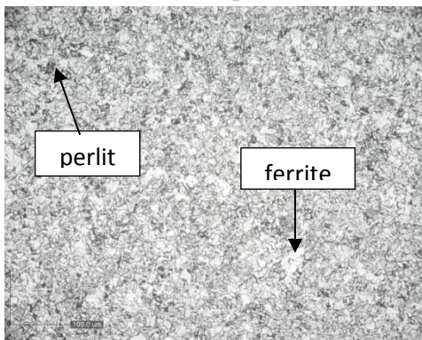
Daerah Struktur Mikro pada sprocket original kondisi As it is (170x pembesaran) Etsa
