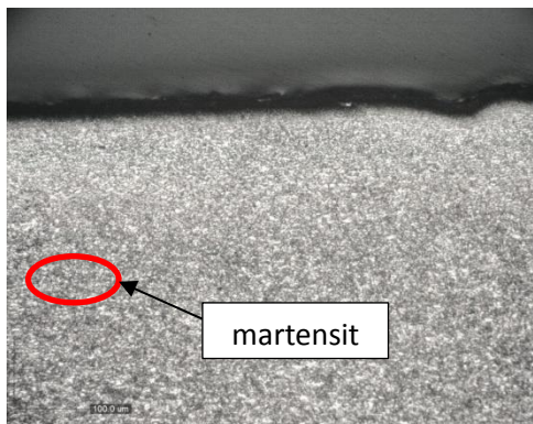
Daerah Struktur Mikro pada sprocket original kondisi As it is (170x pembesaran) Etsa Nital
