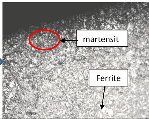
Daerah Struktur Mikro pada sprocket original kondisi As it is (340x pembesaran) Etsa Nital
