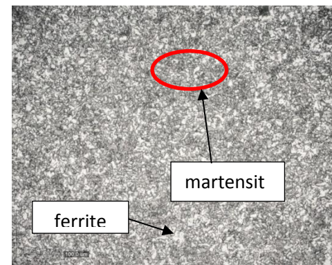
Daerah Struktur Mikro pada sprocket original kondisi As it is (170x pembesaran) Etsa
