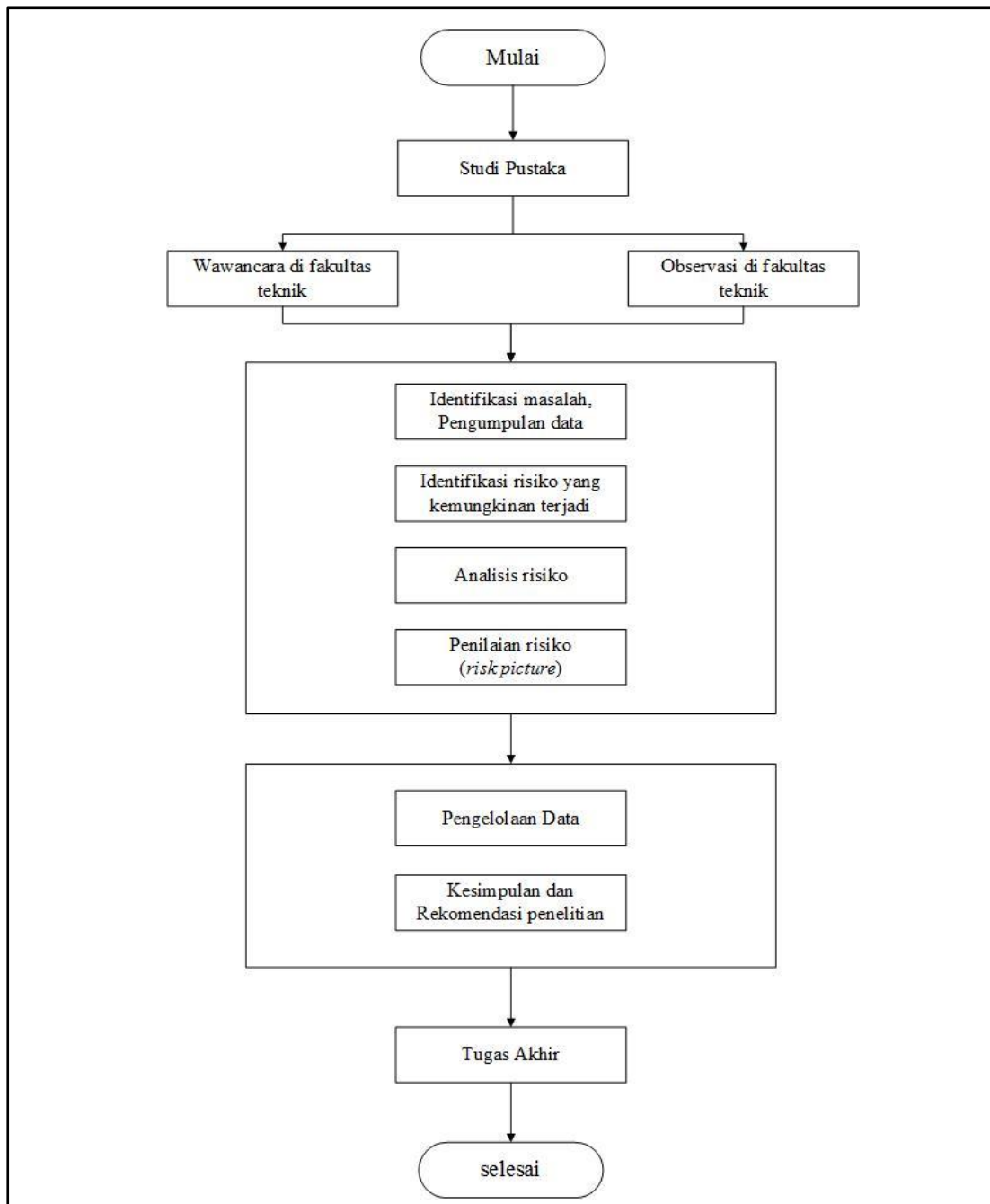
Gambar 1.1 Metodologi Penelitian
