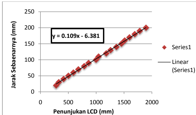
Gambar 4.1 Kurva Penunjukan LCD vs Jarak Sebenarnya
