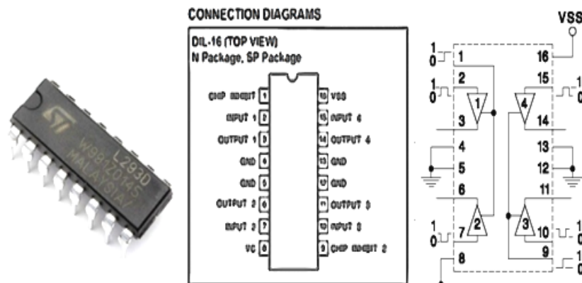
Gambar 2.3 Bentuk dan Simbol IC L293D
