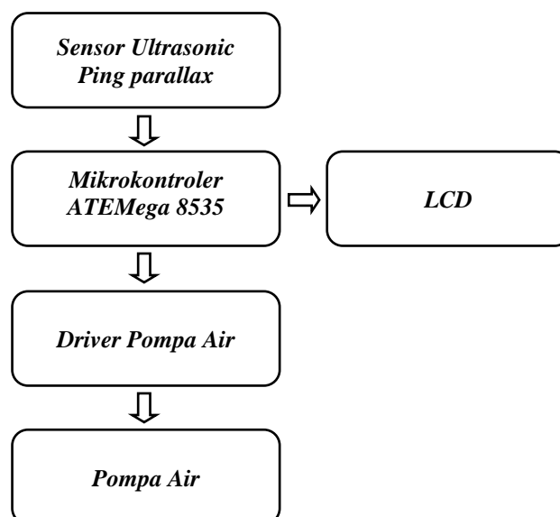
Gambar 3.1 Skema Diagram Blok Rangkaian Penanggulangan Banjir Di Laboratorium Otomasi
