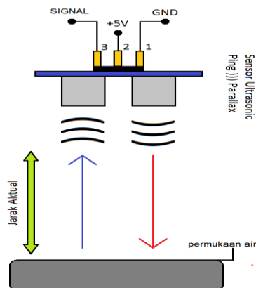
Gambar 3.2 Sensor Ultrasonik Ping Parallax Sebagai Pendeteksi Ketinggian Air di Penampungan
