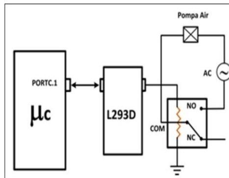
Gambar 3.6 Skematik Rangkaian Driver Pompa Air
