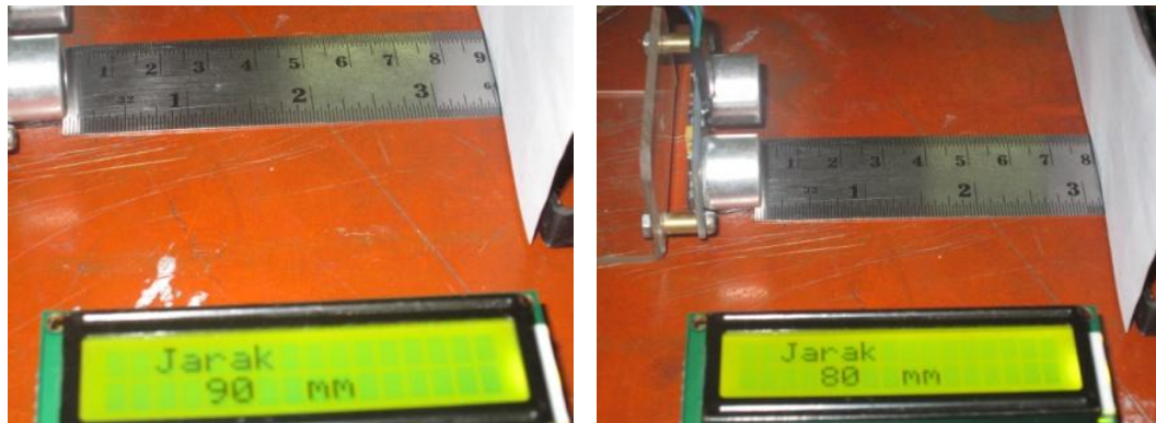
Gambar 4.2 Keakuratan Penunjukan LCD Terhadap Jarak Sebenarnya
