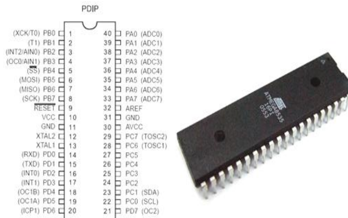
Gambar 2.2 Bentuk IC ATmega8535
