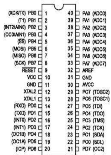
Gambar 3. Konfigurasi PIN ATmega 16
