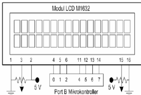
Gambar 5 Rangkaian koneksi LCD dengan Mikrokontroler
