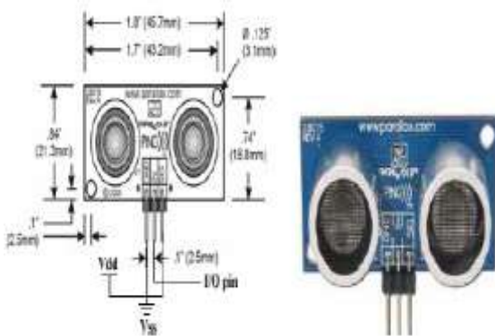
Gambar 2 Bentuk sensor ultrasonik
