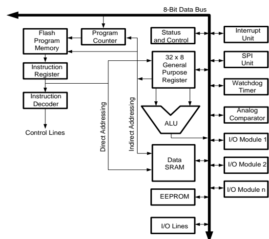
Gambar 4. Arsitektur ATmega 16
