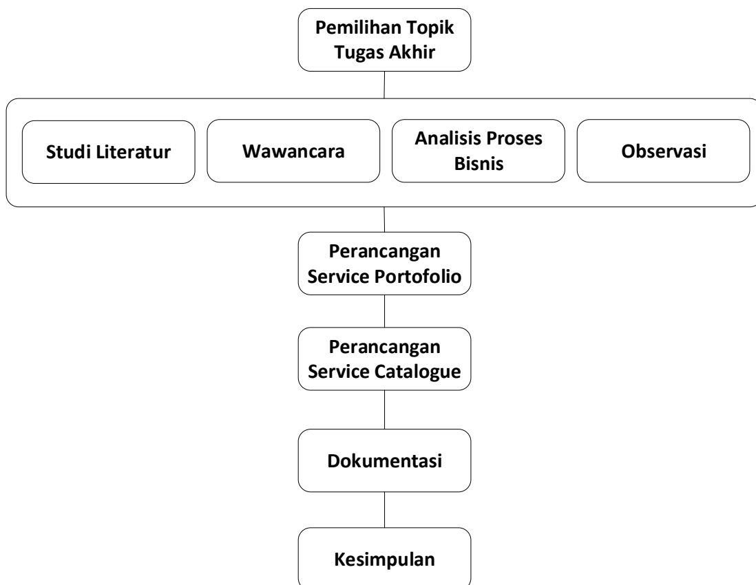
Gambar 1.1 Metodologi Penelitian
